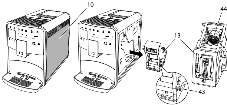
Abb. 23: Brühgruppe ausbauen
